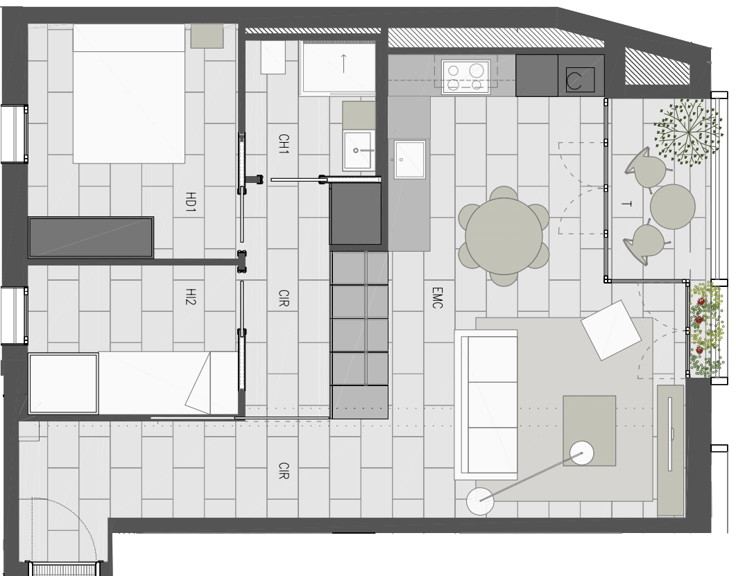
PLANTA BAIXA
