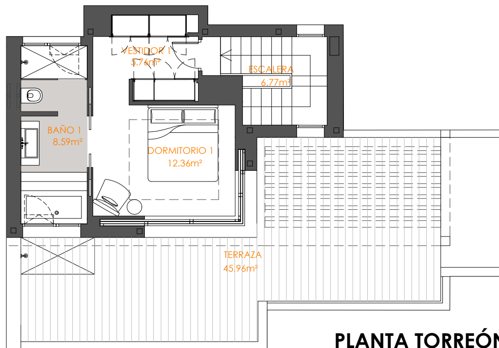
PLANTA SEGUNDA
