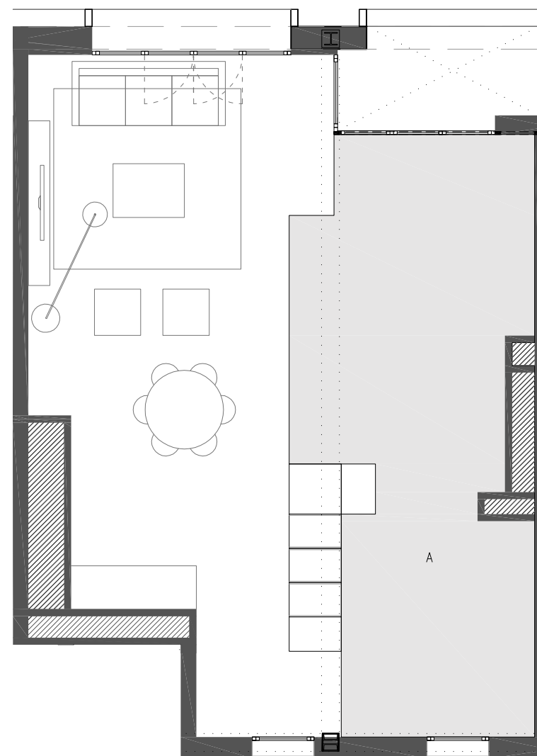
PLANTA ALTELL
