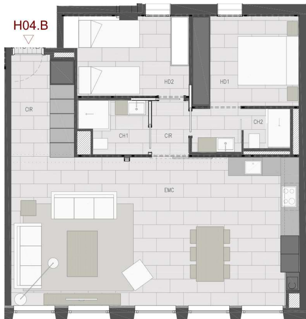
PLANTA BAIXA
