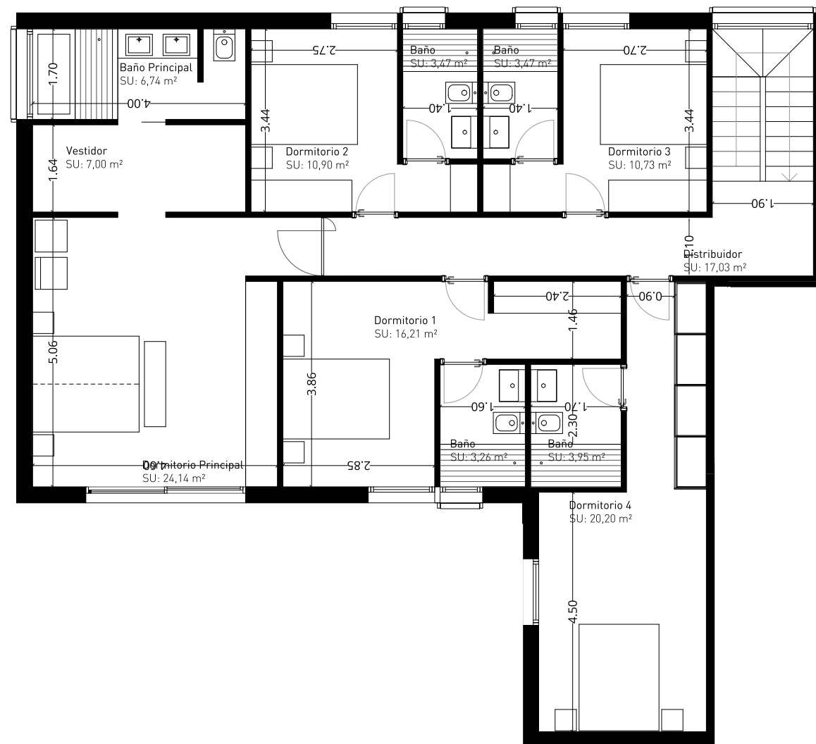
Planta alta
