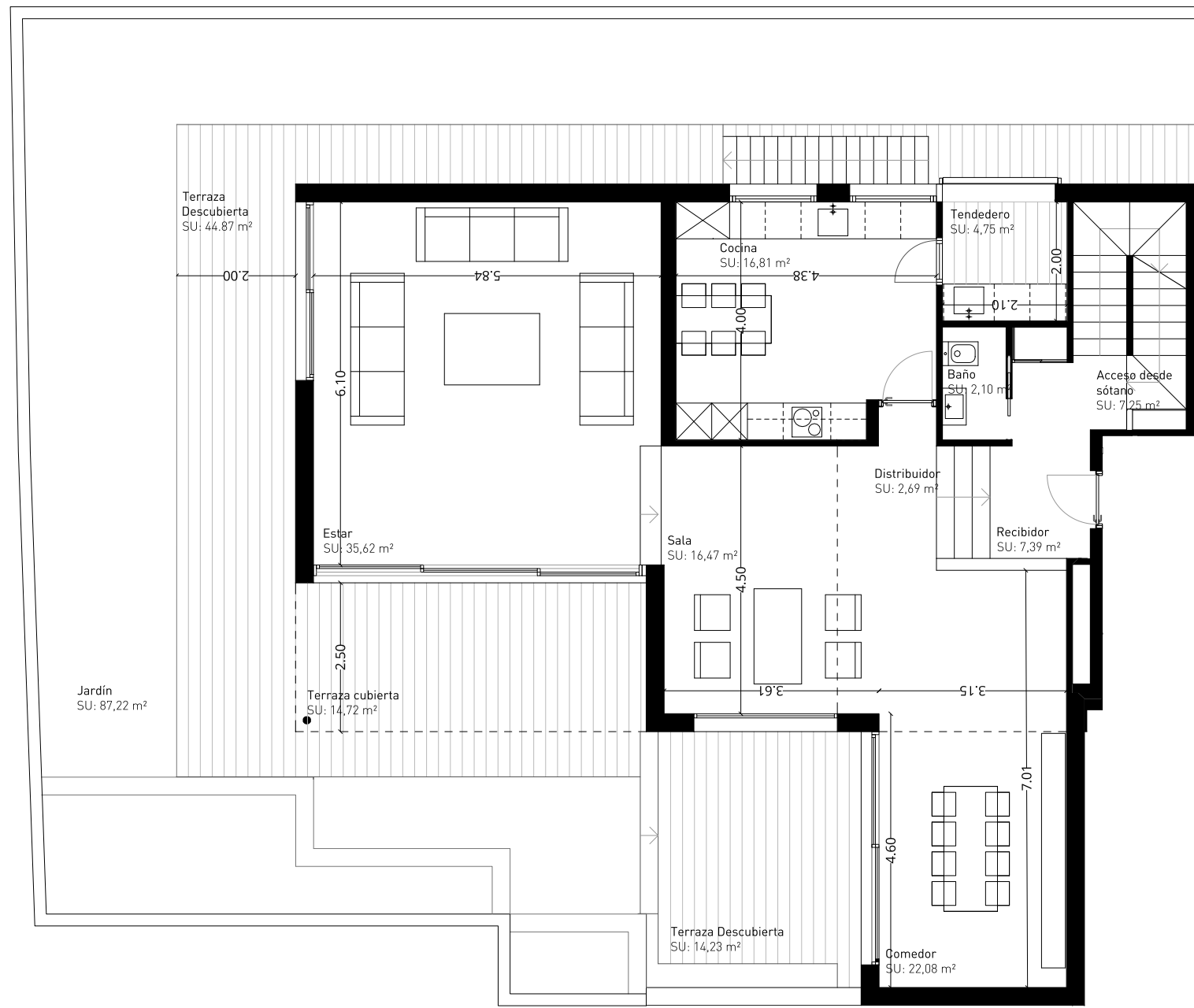
Planta baja
